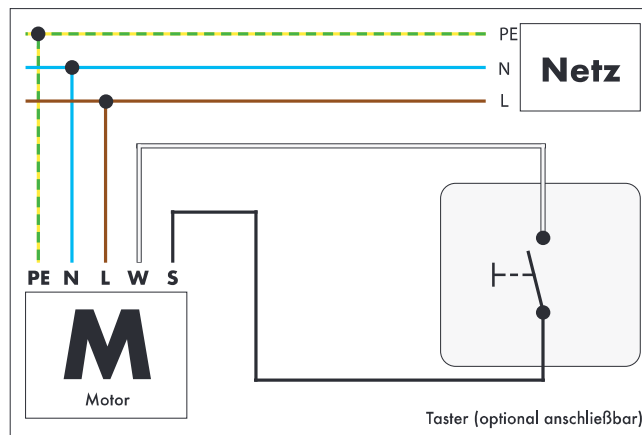
Abb.2: Anschlussschema Art. 140010 - 140050
